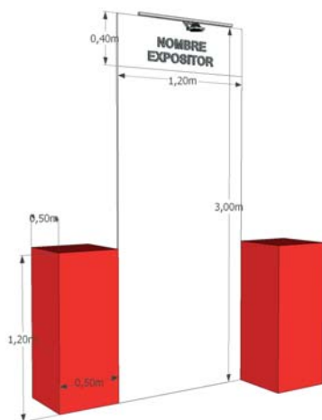
Perspectivas del modelo de stand incluido en la opción de participación Stand Networking
